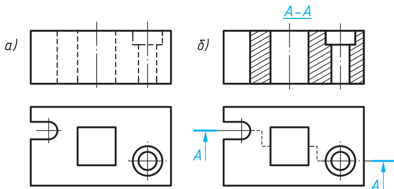
Расми 182. Иҷрои буришгоҳи мураккаб: а – ду намуни маснуот; б – акси буришгоҳи мураккаб
