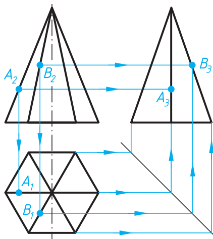
Расми 94. Сохтани проексияи нуқтаи дар теғаи пирамида хобида
