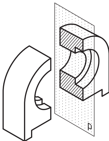
Расми 178. Ҳосил кардани буришгоҳи паҳлуй
