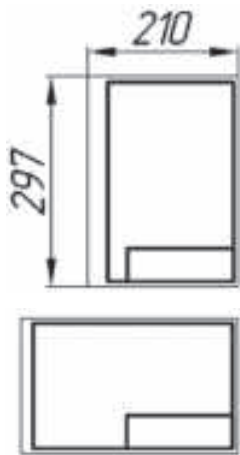
Расми 19. Ороиши варақи нақшакашӣ
