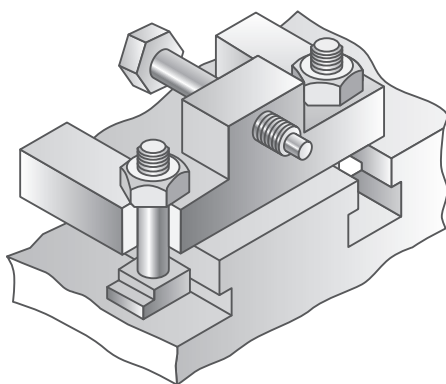
Расми 230. Нақша ва тасвири аёнии таъя
