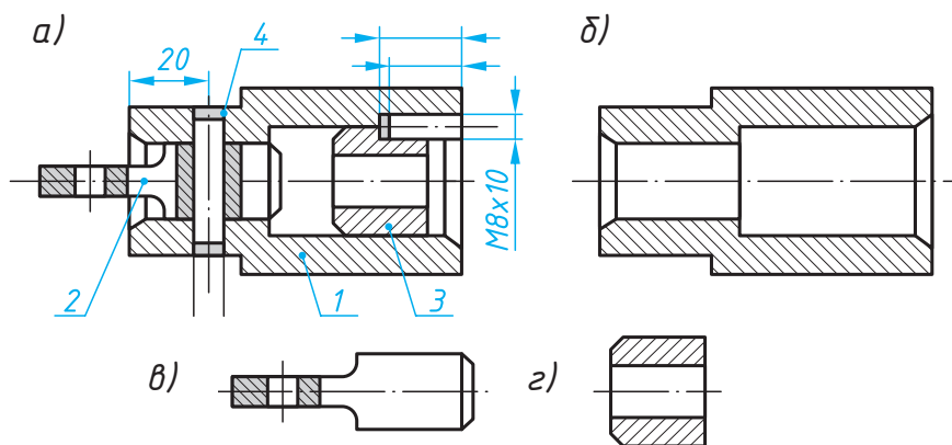
Расми 242. Нақшаи васлияи маснуот ва ҷузъҳои он
