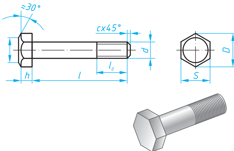
Расми 218. Болти саракаш шашрӯя
