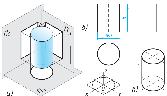
Расми 82: а — проекциясозӣ; б — нақшаи устувона дар системаи проексияҳои росткунҷа; в — проексияи изометрии устувона
