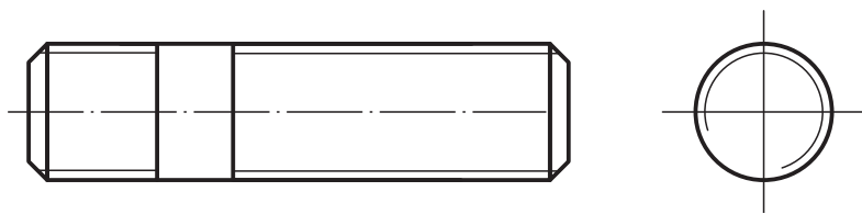
Расми 214. Тасвири печ дар санҷоқ
