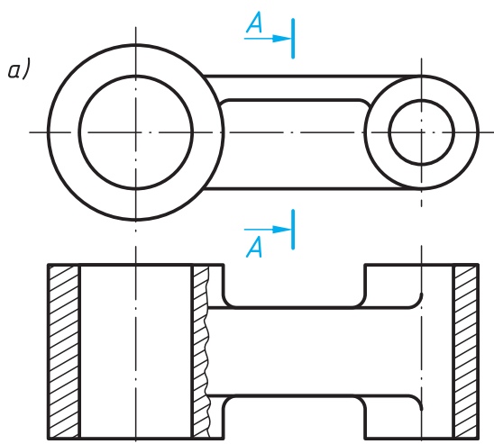
Расми 162. Тана: а — тасвири буридашудаи (нимаи) қисм; б — тасвири аёни
