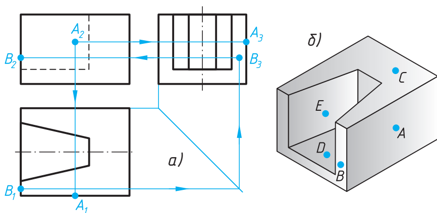
Расми 96. Сохтани проексияҳои нуқтаҳое, ки дар сатҳи ҷисм ҷойгиранд
