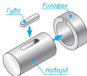
Расми 222. Тасвирҳои аёнии чузъҳои пайвасти гувагӢ
