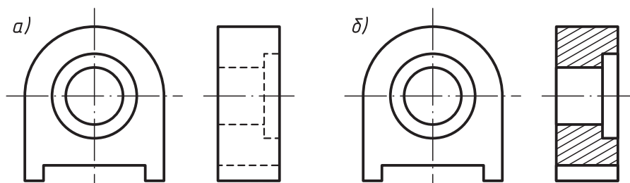
Расми 178. Ҳосил кардани буришгоҳи паҳлуй
