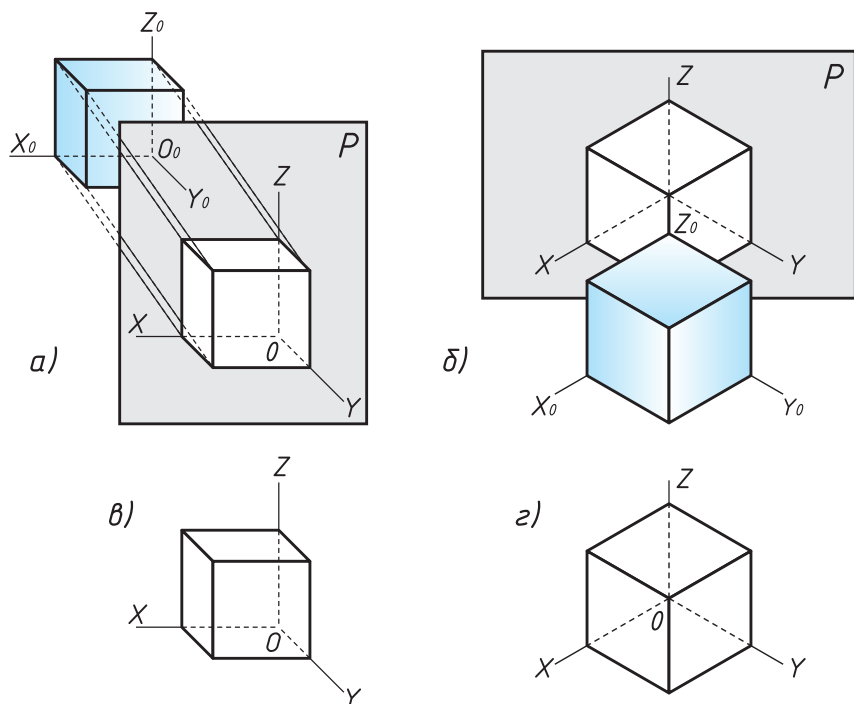
Расми 59. Ҳосил кардани проексияи аксонометрӣ: а, в — фронталӣ диметрӣ; б, г — изометрӣ
