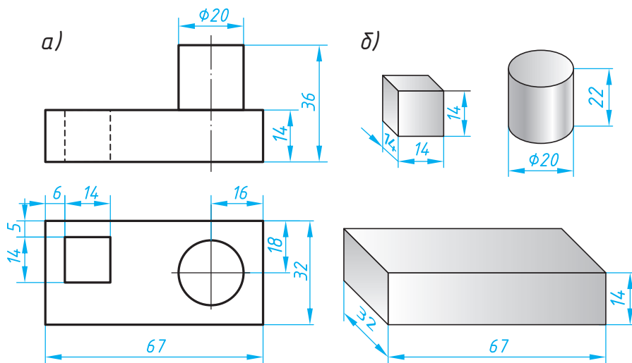
Расми 121. Тарзи андозагузорӣ
