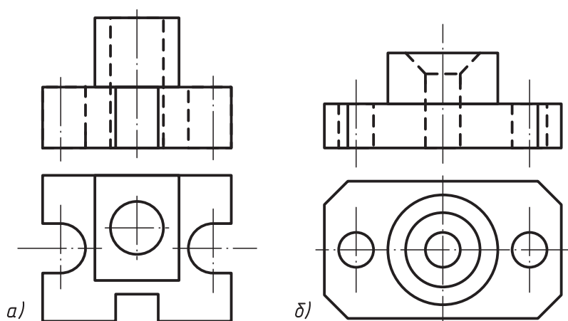
Расми 194. Супориш барои машқ
