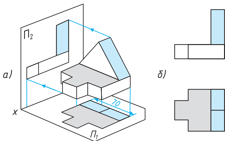
Расми 44: а — сохтани проексияи ҷисм дар ду ҳамвори проексияҳо; б — нақшае, ки аз ду проексия иборат аст
