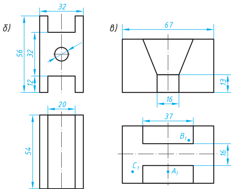
Рисми 116. Супориш барои машқ
