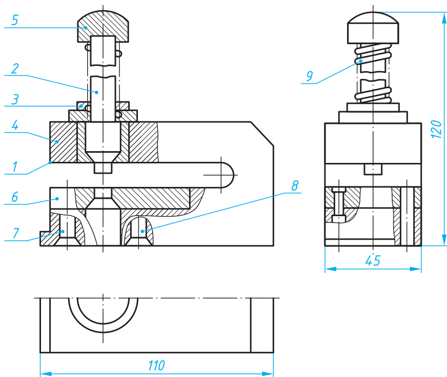
Расми 241. Нақшаи ҷиҳози сӯрохкунанда
