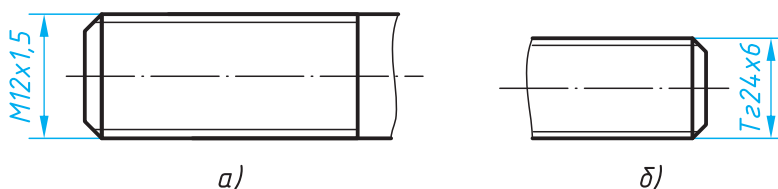
Расми 216. Ишорати печ
