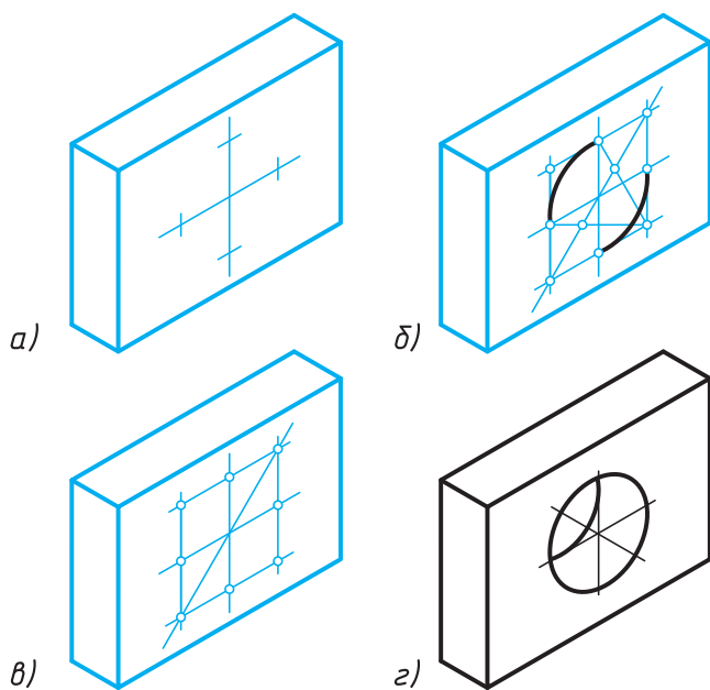
Расми 68. Сохтани проексияҳои аксонометрии чисмҳое, ки сатҳҳои мудаввар доранд
