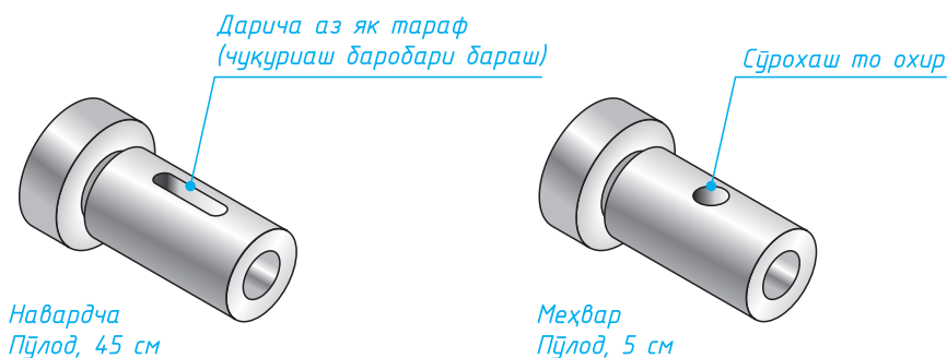
Расми 173. Супориш барои машқ
