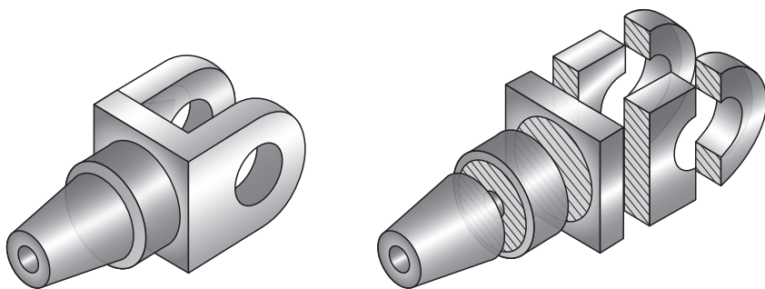
Расми 75. Таҳлили геометрии шакли маснуот
