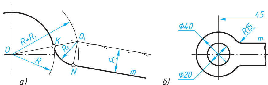
Расми 136. Пайвастанӣ камони давра бо хатти рост
