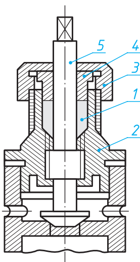
Расми 234. Нақша барои хондан
