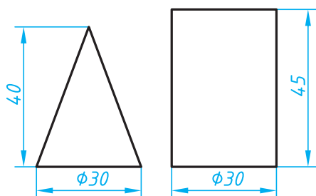
Расми 84. Истифодаи аломати шартӣ, ки шакли чисмҳоро муайян месозад
