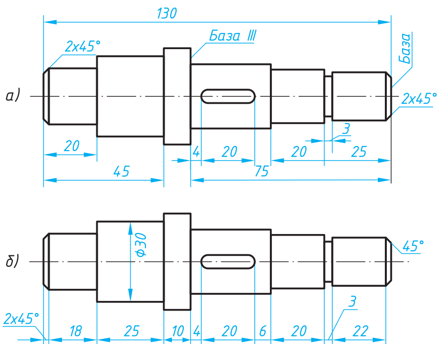
Расми 122. Тарзҳои андозагузорӣ
