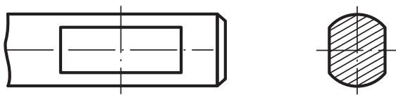
Расми 168. Тасвири буриши симметрие, ки дар давоми хатти буриш ҷойгир аст
