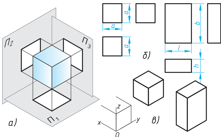
Расми 77: а — проекциясозӣ, б — нақшаҳои мукааб ва параллелепипед; в — проексияи изометрии мукааб
