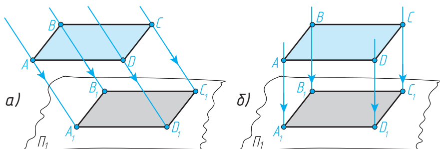
Расми 40: а — проексиясозии каҷкунҷа, б — проексиясозии росткунҷа
