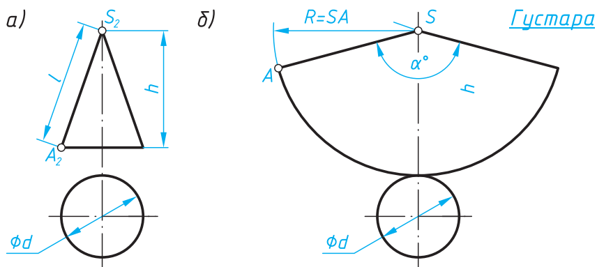
Расми 142. Сохтани нақшаи густараи сатҳи махрут: а — ду намуни махрут; б — густараи сатҳ
