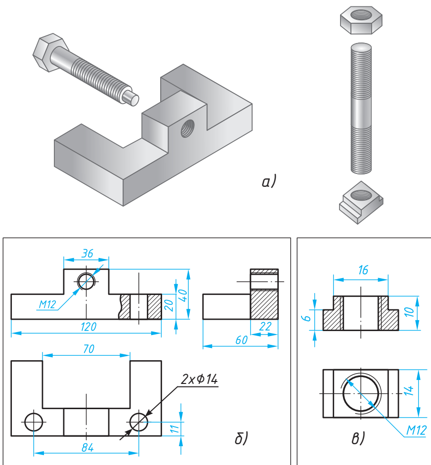
Расми 237. Тасвири аёни ва нақшаҳои чузъҳои така
