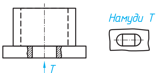
Расми 52. Намуди ҷузъй
