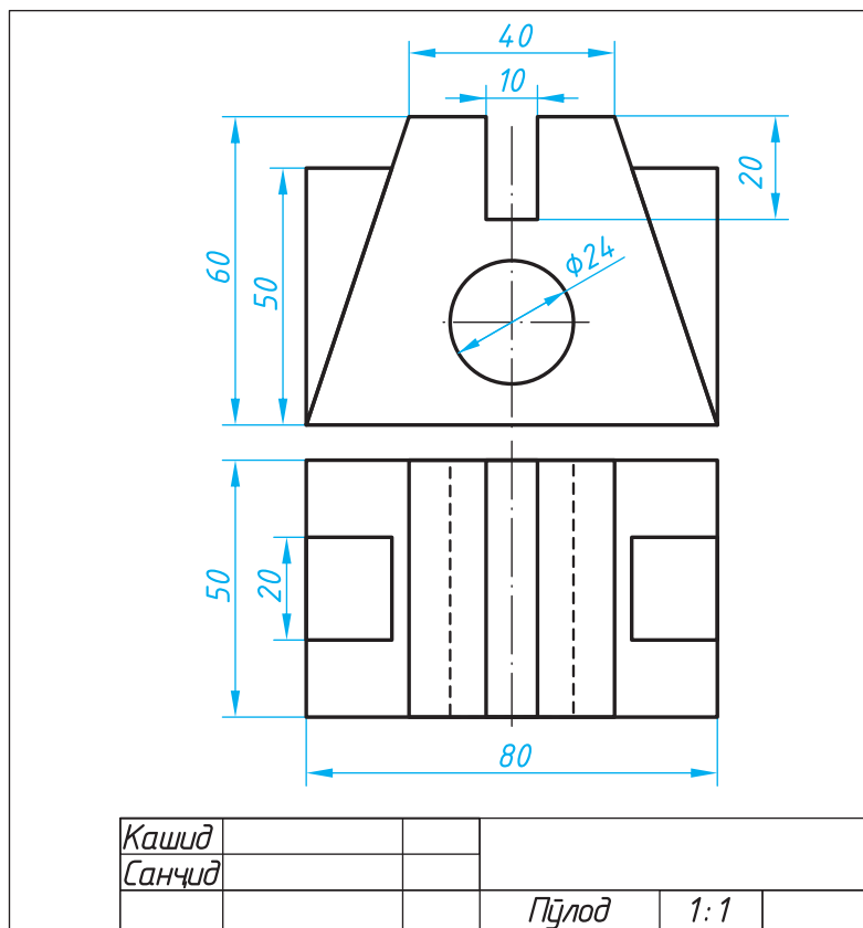
Расми 146. Супориш барои машқ
