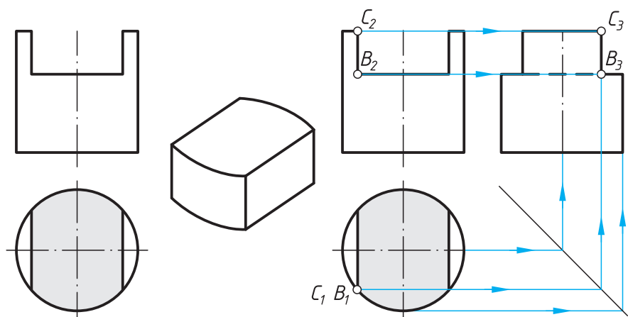
Расми 110. Сохтани проексияҳои комаи ҷисм
