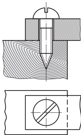
Расми 229. Супориш барои машқ
