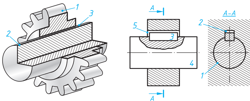
Расми 227. Супориш барои машқ
