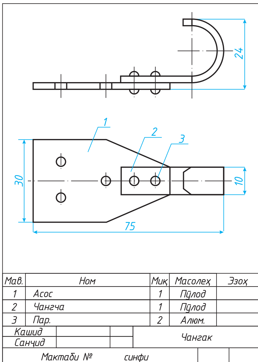
Расми 7. Нақшаи васлия
